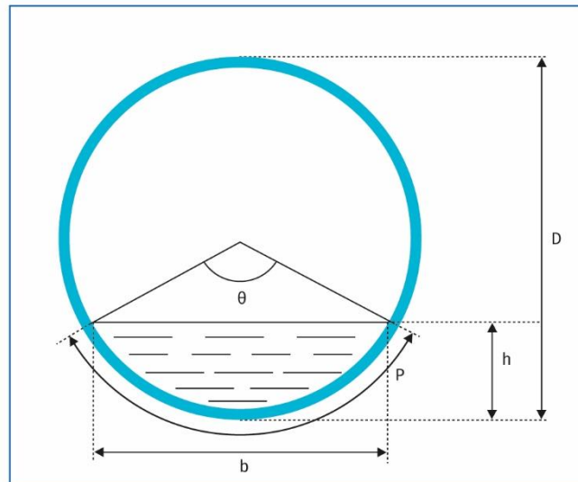
Figure 34 : Paramètres de Pomeroy
