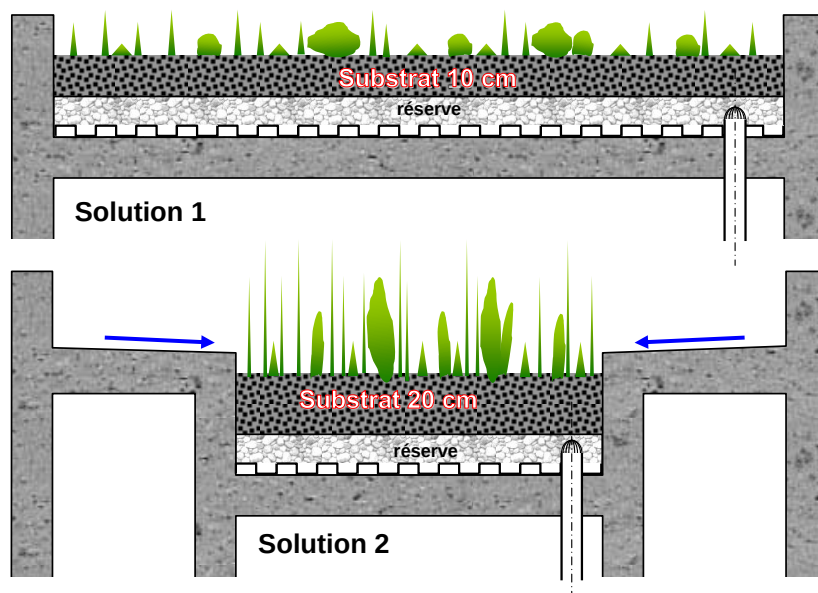
Figure 36 : Schémas illustrant le principe d'équivalence
