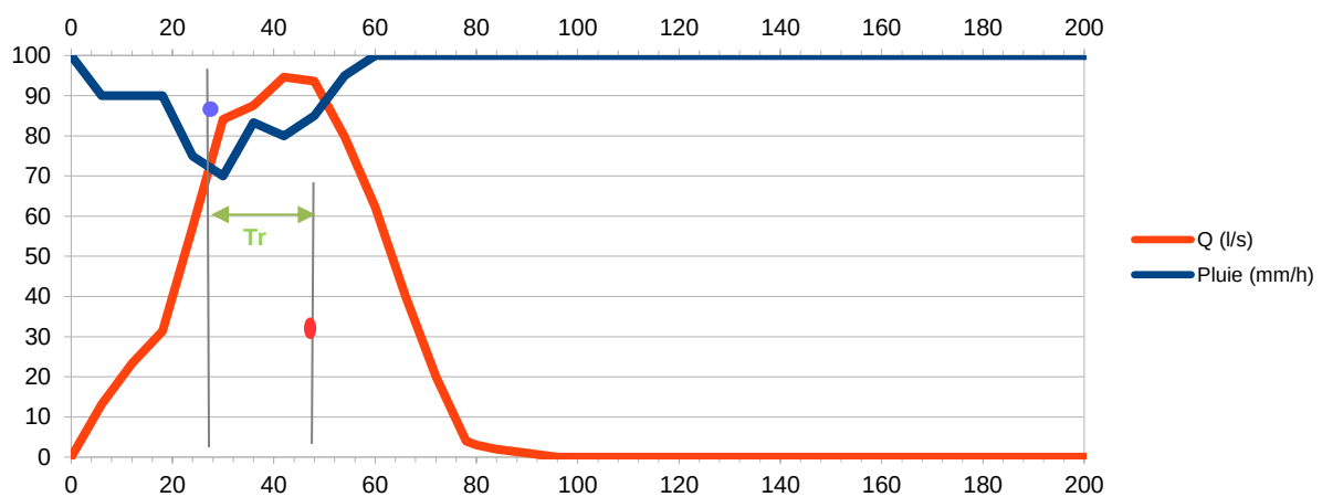
Figure 22 : Estimation graphique de t_r
