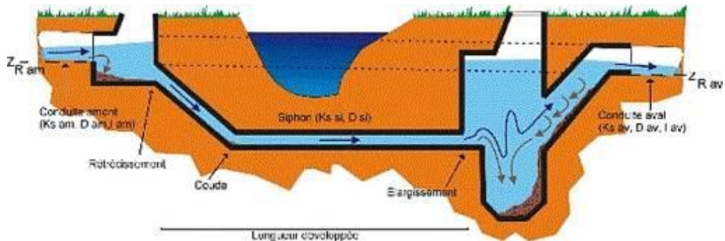
Figure 123 : Composants d'un siphon
