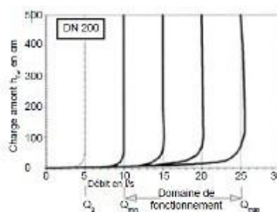
Figure 127 : Exemple de courbe de débit d'un régulateur à flotteur (UFT France)
