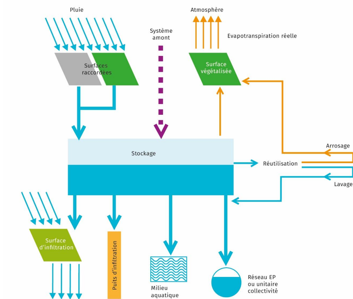
Figure 4 : Schéma de principe montrant les différentes sources d'eaux de ruissellement et les exutoires possibles moyennant un stockage tampon
