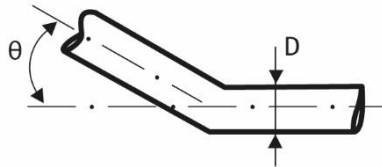
Figure 125 : Paramètres de calcul des pertes de charge dans un coude à angle vif
